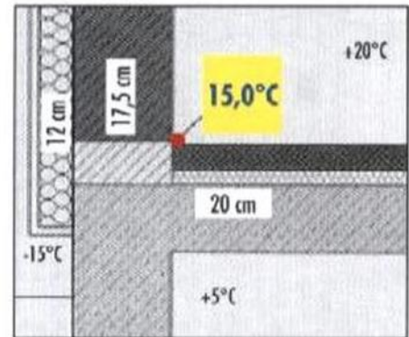
Con ISOMUR® la temperatura ne l'angolo basso evita la formazione di condensa
