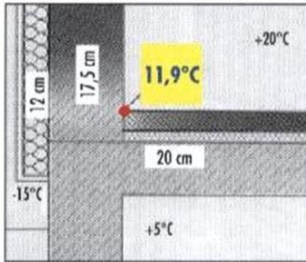
Situazione standard rischio formazione condensa
